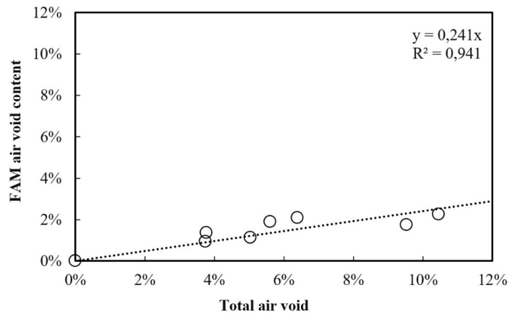
Figure 14. Correlation between total AC AV and FAM AV contents
